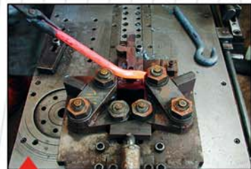
Presses horizontales HYDROIL de 10 à 35T Cintrage maxi 50mm
